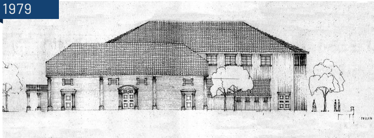
Comediehuset Ugland & Thornes foreslåtte teaterrombygging av Otterslands lager, med en rekonstruksjon av Comediehuset i front. 1979 Arkitekter: Arkitektkontoret Kjell Jensen (Drange & Aanensen). Digitalisert: Mona Hauglid.
